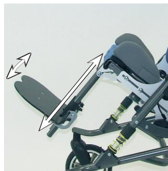
réglage en hauteur et inclinaison du repose pieds
